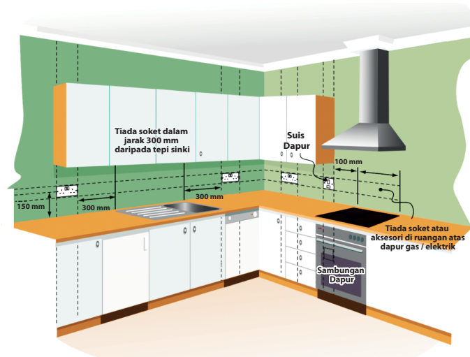
Rajah 6.15: Jarak Selamat Antara Soket Alir Keluar dan Sinki Dapur Serta Jarak Ketinggian Selamat Antara Soket Alir Keluar dan Kabinet Dapur
