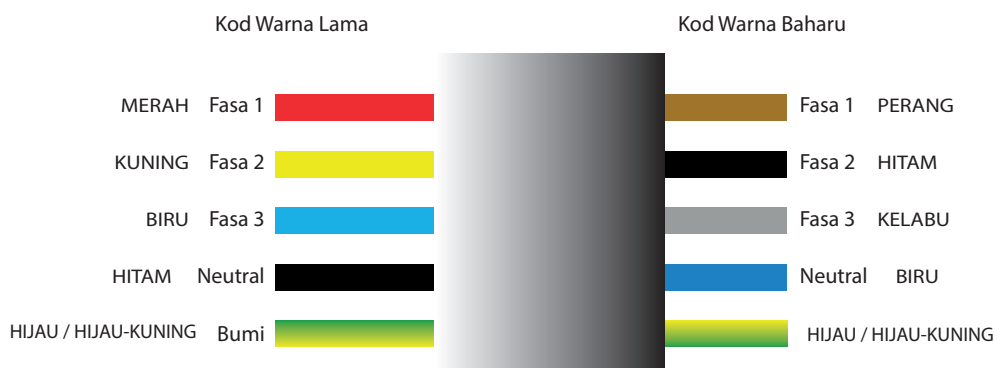
Rajah 8.1: Perbandingan Kod Warna Lama dan Baharu Merujuk IEC 60445
