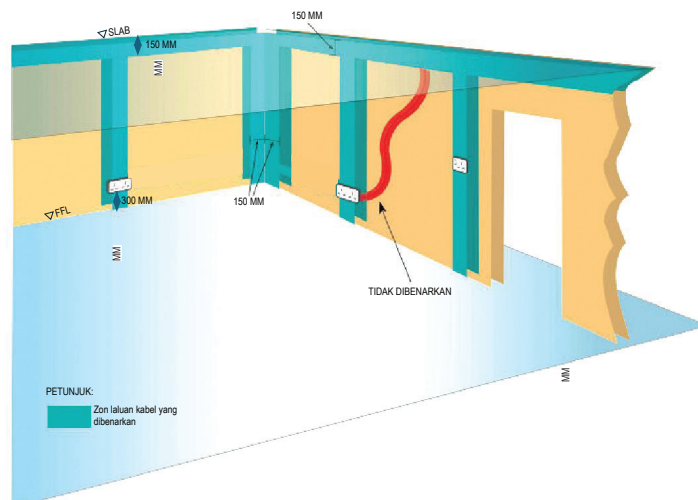
Rajah 6.16: Zon Laluan Kabel Pendawaian yang Dibenarkan
